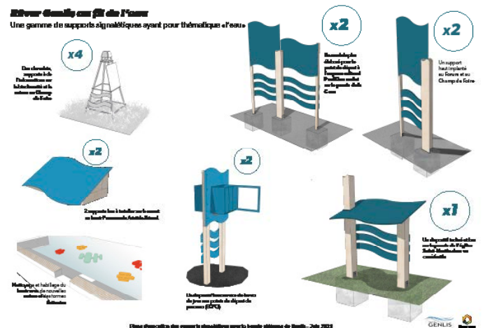
Dessins d'exécution des supports signalétiques sur chaque site (3D, détails techniques et découpage des actions)
